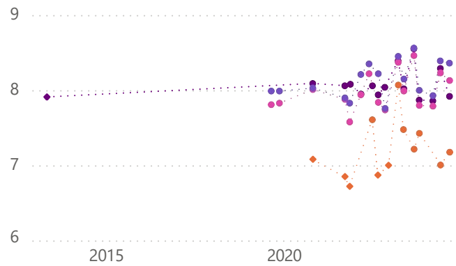
pH (Lab)
